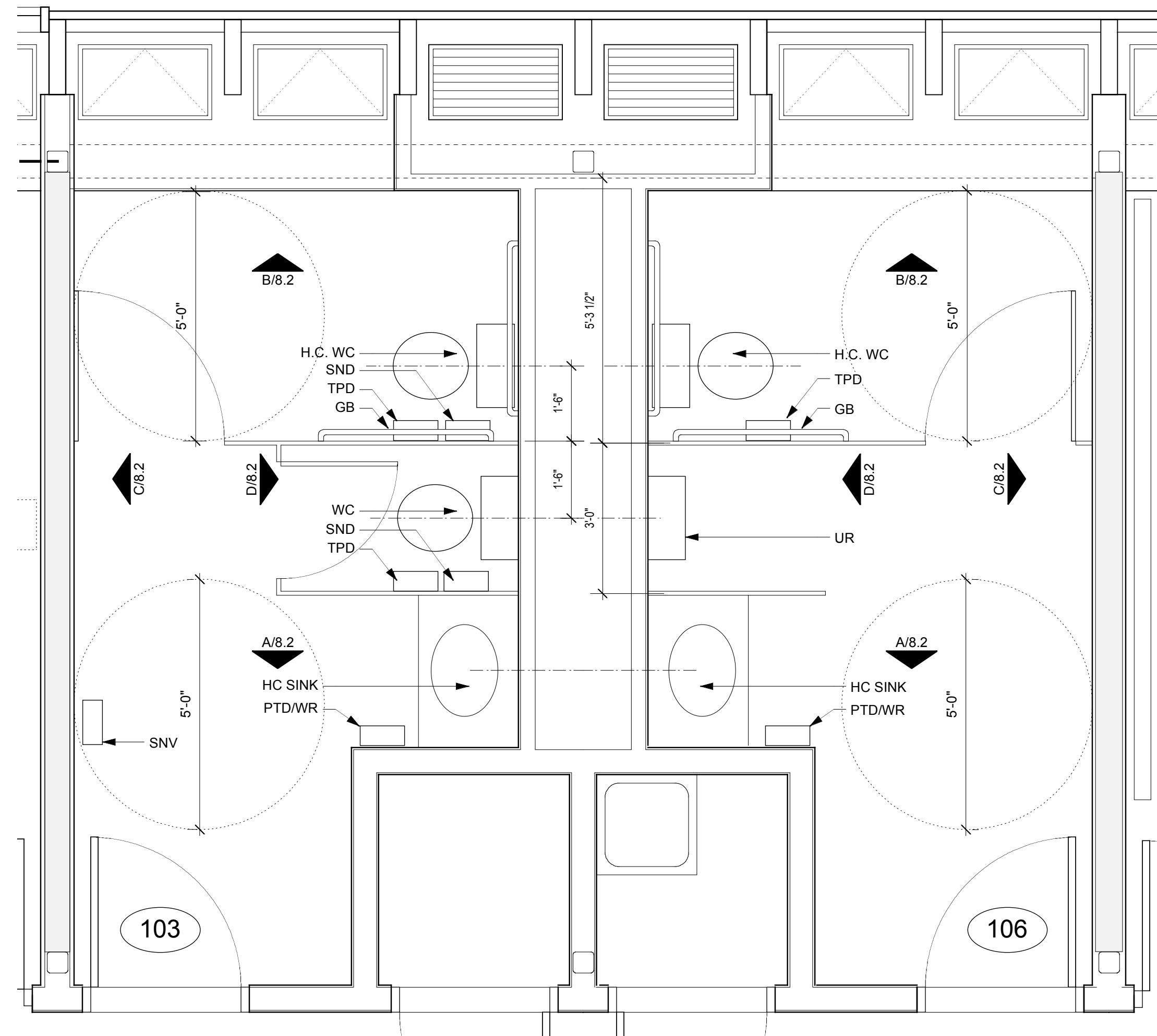
1 TOILET PLANS 1/4"=1'-0"
